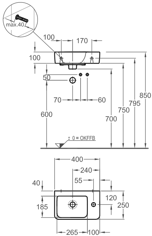
Renova Nr.1 Comprimo Handwaschbecken 400, Becken links mit Hahnloch Mod.-Nr. 27 61 40 06.02.2013/Th
